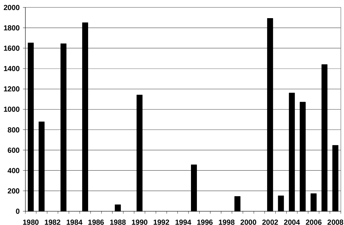
Figuur 5. Aantallen Zilverplevieren op Texel in september, op basis van de tussen 1980 en 2008 in deze maand uitgevoerde wad- en watervogeltellingen
